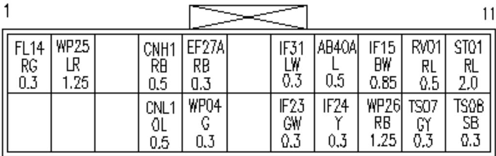
接仪表板电线束总成 FB-IP2
