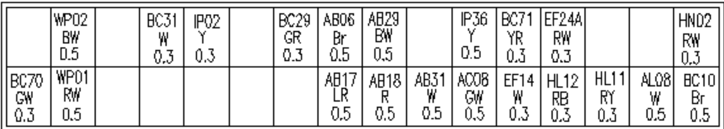
接仪表板电线束总成 FB-IP1
