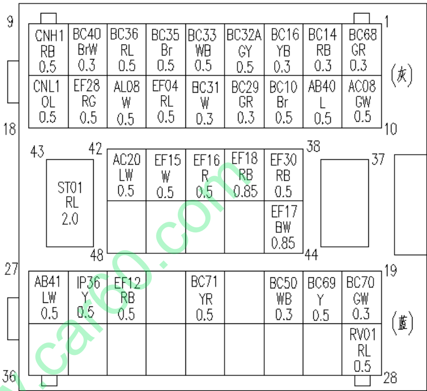
接机舱电线束总成 EN-FB1
